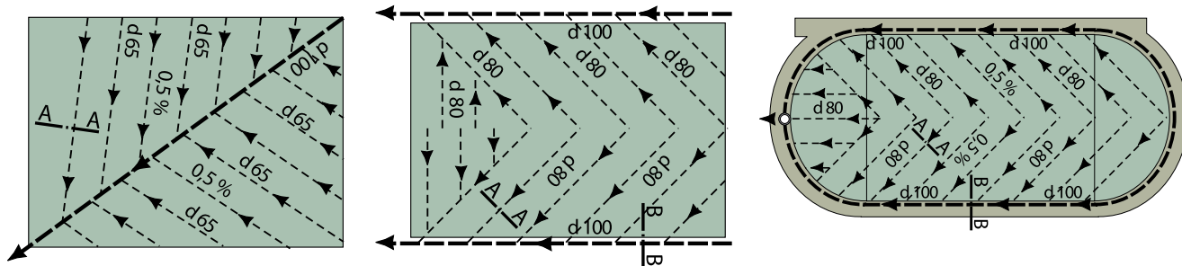
a - příklad návrhu drenáže
