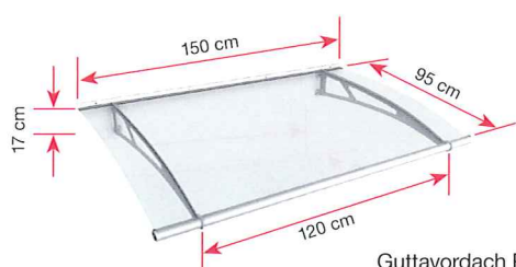
Guttavordach PT/L(W) 150
