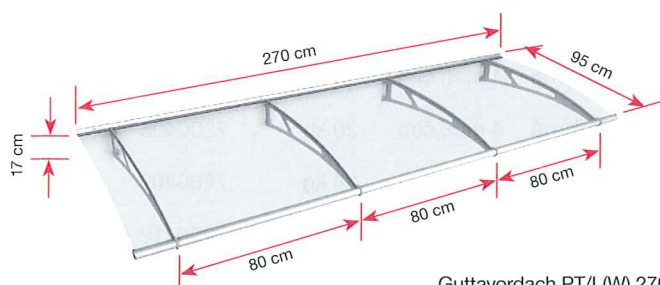
Guttavordach PT/L(W) 270
