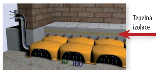
9 Výstavba nebo montáž nášlapné vrstvy podlahy, včetně uložení rozvodů vody, elektřiny a podlahového vytápění.
